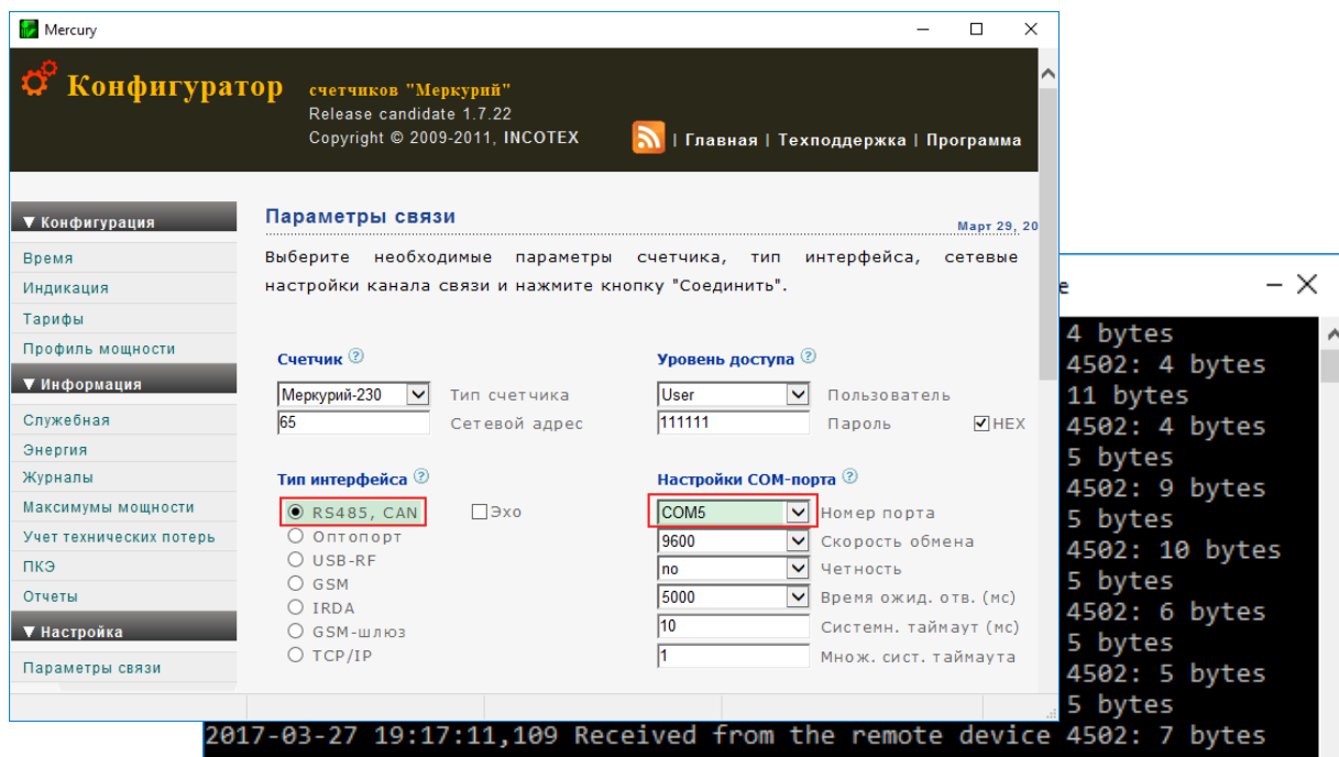
Рис. 17. Настройка подключения «Конфигуратор Меркурий» к серверу M2M24 (COM-порт).
