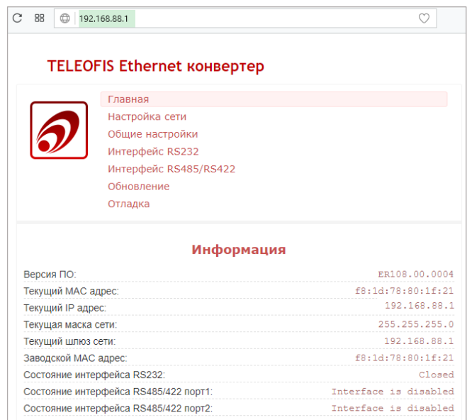
Рис. 5. Web-интерфейс для настройки конвертера ER.
