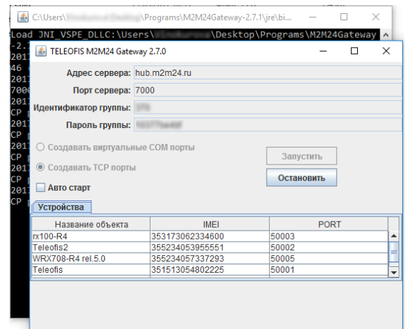
Рис. 10. M2M24 Gateway. Главное окно приложения.
