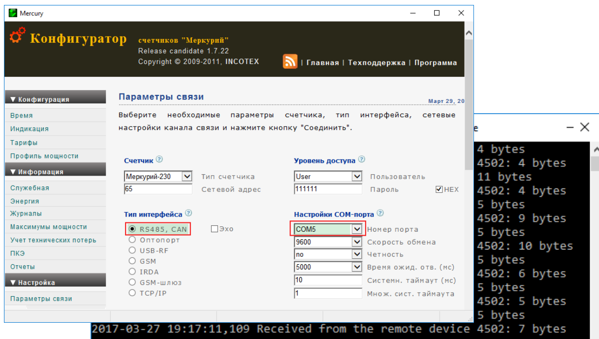
Рис. 15. Настройка подключения «Конфигуратор Меркурий» к серверу M2M24 (COM-порт).
