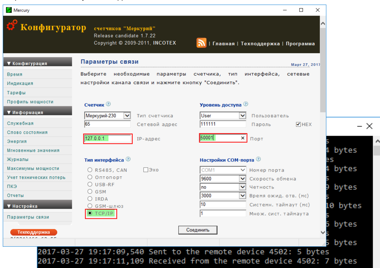
Рис. 12. Настройка подключения «Конфигуратор Меркурий» к серверу M2M24 (TCP-порт)
