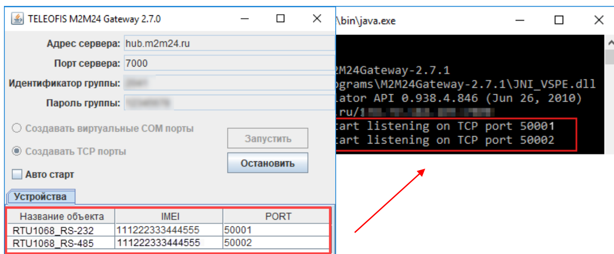
Рис. 11. Запуск шлюза M2M24 Gateway.
