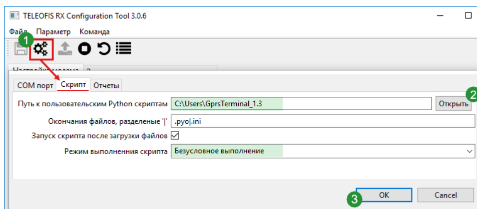
Рис. 8. Загрузка настроек скрипта GPRS Terminal в программу.
