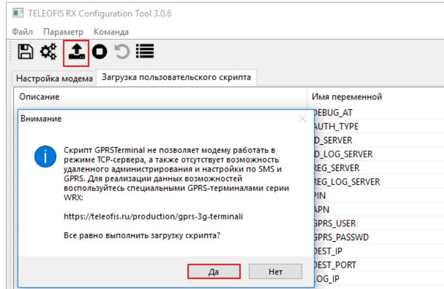
Рис. 10. Окно уведомления при загрузке скрипта GprsTerminal .
