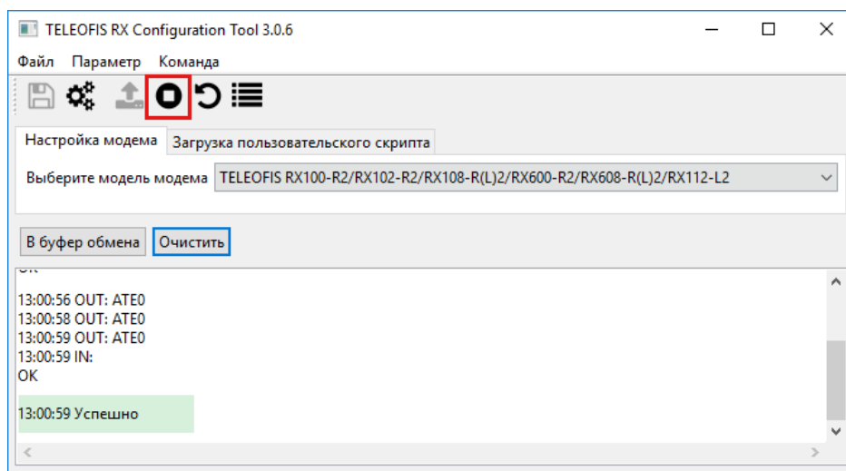
Рис. 7. Остановка скрипта в программе RX Configuration Tool.
