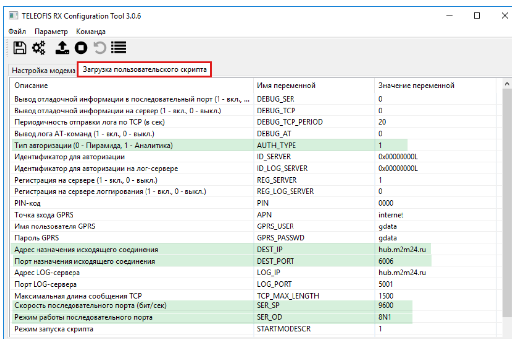
Рис. 9. Отображение настроек скрипта GprsTerminal в RX Configuration Tool.
