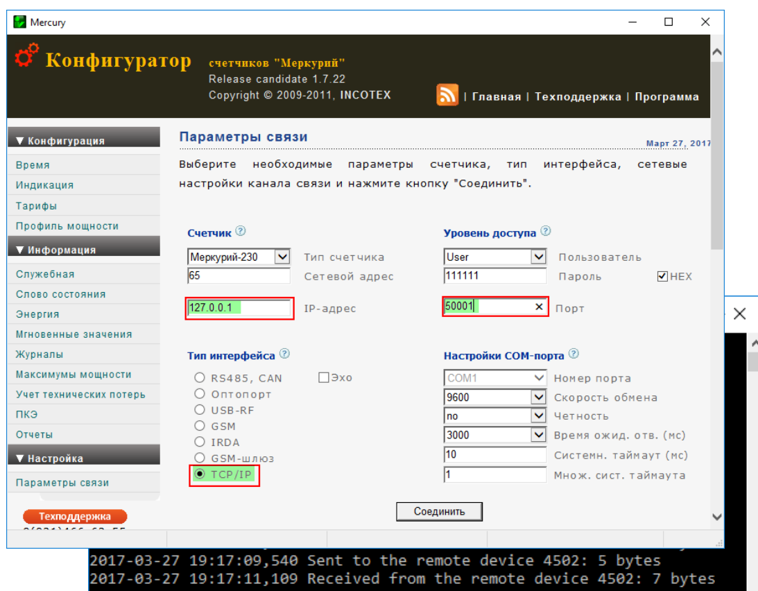
Рис. 17. Настройка подключения «Конфигуратор Меркурий» к серверу M2M24 (TCP-порт).
